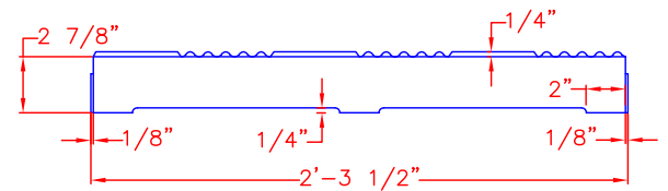
END ELEVATION
